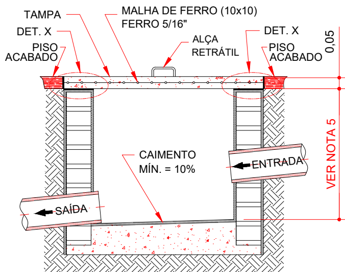
CORTE A-A
