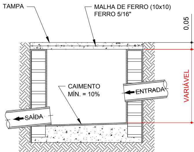
CORTE A-A
