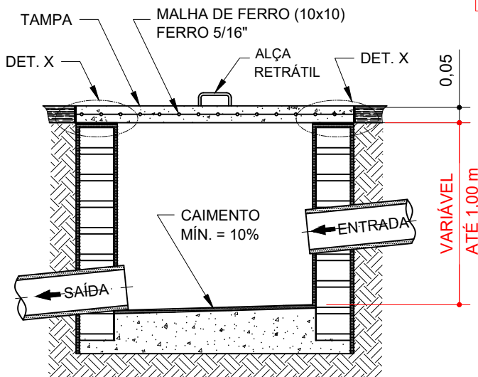
CORTE A-A
