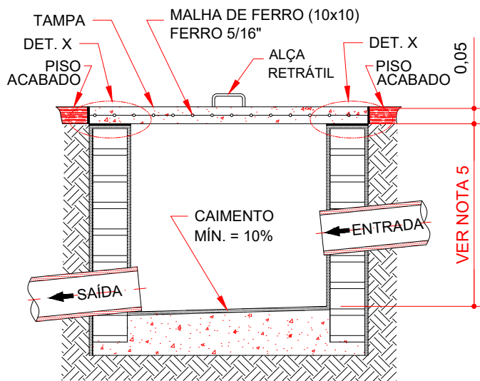
CORTE A-A
